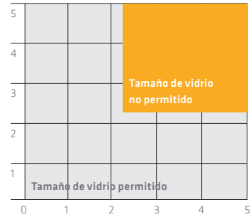
Fig. 3a: Tamaño de elemento SG factible con la Sikasil® SG-500, dimensión de la junta SG: 12 mm x 6 mm; carga de viento: 1.50 kPa; carga muerta soportada
