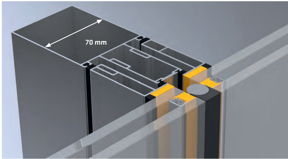
Fig. 3b: Bajo las mismas condiciones que en la fig. 3a los elementos de fachada pueden ser de mayor dimensión con la Sikasil® SG-550. Del mismo modo la altura de la junta para el mismo tamaño de elemento puede ser un 30% más pequeña, consiguiendo un ahorro del volumen total de la junta incluso del 60%.
