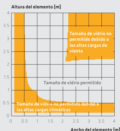
Fig.2 Las cargas climáticas y las cargas de viento son relevantes en el cálculo de la altura del sellador del doble acristalamiento
