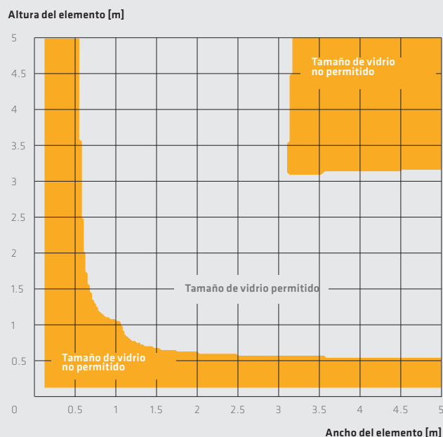
Fig. 4b: Bajo las mismas condiciones de la Fig. 4a las unidades doble/triple acristalamiento pueden ser de mayor tamaño con la Sikasil® IG-25 HM Plus. Del mismo modo la altura de la junta para el mismo tamaño de elemento puede ser un 25% más pequeña.
