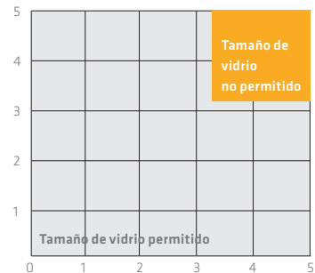
Fig. 3b: Bajo las mismas condiciones que en la fig. 3a los elementos de fachada pueden ser de mayor dimensión con la Sikasil® SG-550. Del mismo modo la altura de la junta para el mismo tamaño de elemento puede ser un 30% más pequeña, consiguiendo un ahorro del volumen total de la junta incluso del 60%.
