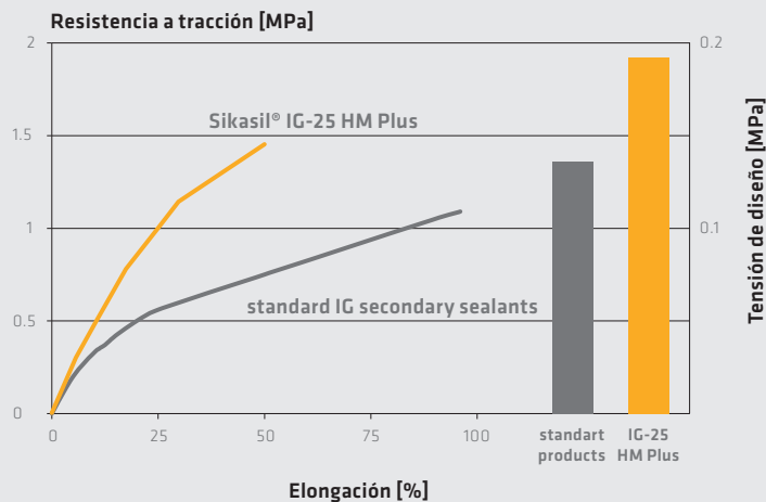
Fig. 2: Comparación de la curva tensión - deformación y la resistencia de diseño de la Sikasil® IG-25 HM Plus con los productos IG estándares.
