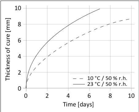
Diagrama 1: Velocidad de curado del Sikaflex®-221
